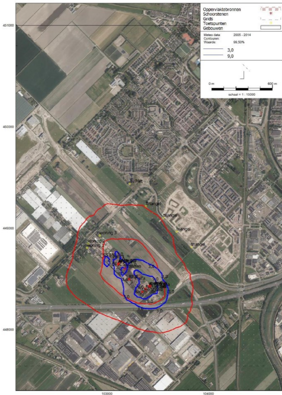
Figuur d Geurcontouren van 3 en 9 ou_E/m^3 als 99,5-percentielwaarde als gevolg van Waddinxveense Groenrecycling Wagro BV in de vergunde en toekomstige situatie - worst case ( 2.500\ ou_E/m^3 )
