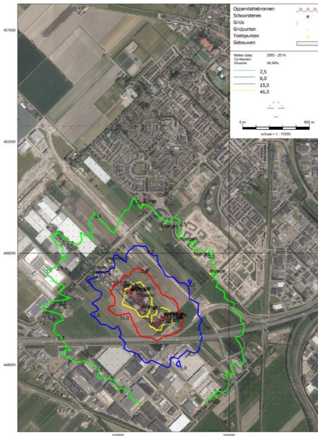
Figuur j Geurcontouren van 2,5; 7,5; 15 en 45 ou_E/m^3 als 99,99-percentielwaarde als gevolg van Waddinxveense Groenrecycling Wagro BV in de toekomstige situatie – worst case ( 2.500\ ou_E/m^3 )
