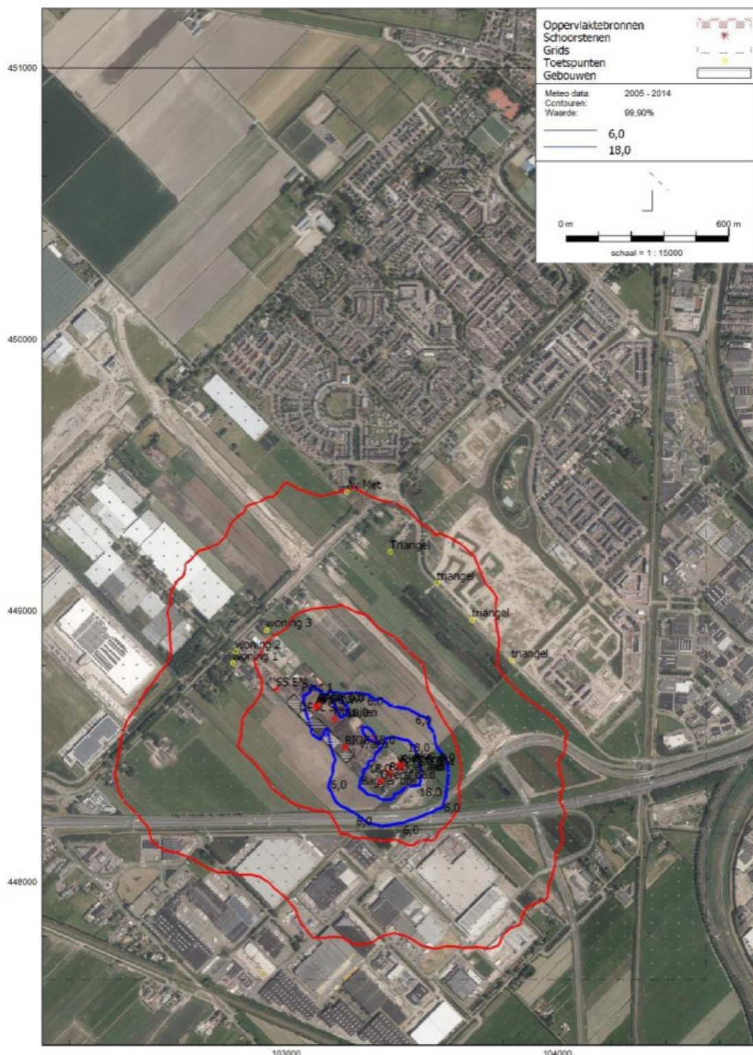
Figuur g Geurcontouren van 6 en 18 ou E /m 3 als 99,9-percentielwaarde als gevolg van Waddinxveense Groenrecycling Wagro BV in de vergunde en toekomstige situatie – best case (1.000 ou E /m 3 )
