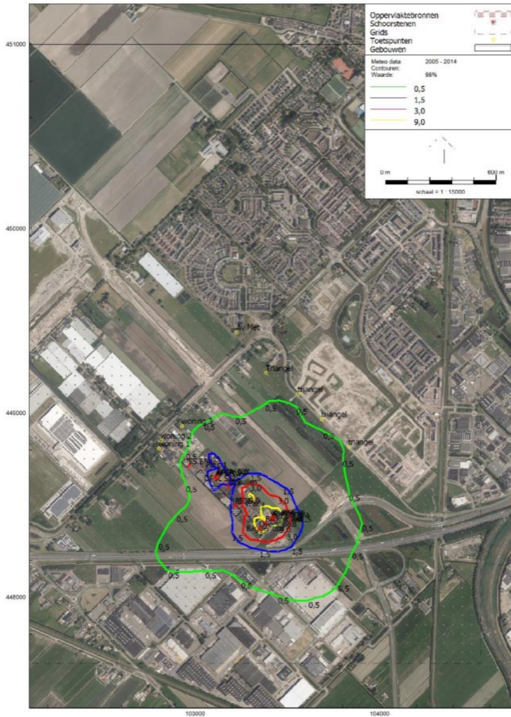
Figuur i Geurcontouren van 0,5; 1,5; 3 en 9 ou_E/m^3 als 98-percentielwaarde als gevolg van Waddinxveense Groenrecycling Wagro BV in de toekomstige situatie – best case ( 1.000\ ou_E/m^3 )
