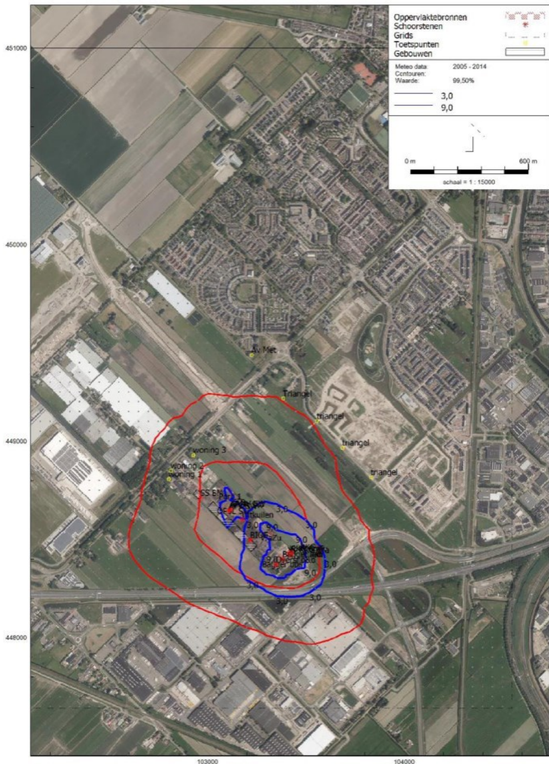
Figuur e Geurcontouren van 3 en 9 ou E /m 3 als 99,5-percentielwaarde als gevolg van Waddinxveense Groenrecycling Wagro BV in de vergunde en toekomstige situatie - best case (1.000 ou E /m 3 )
