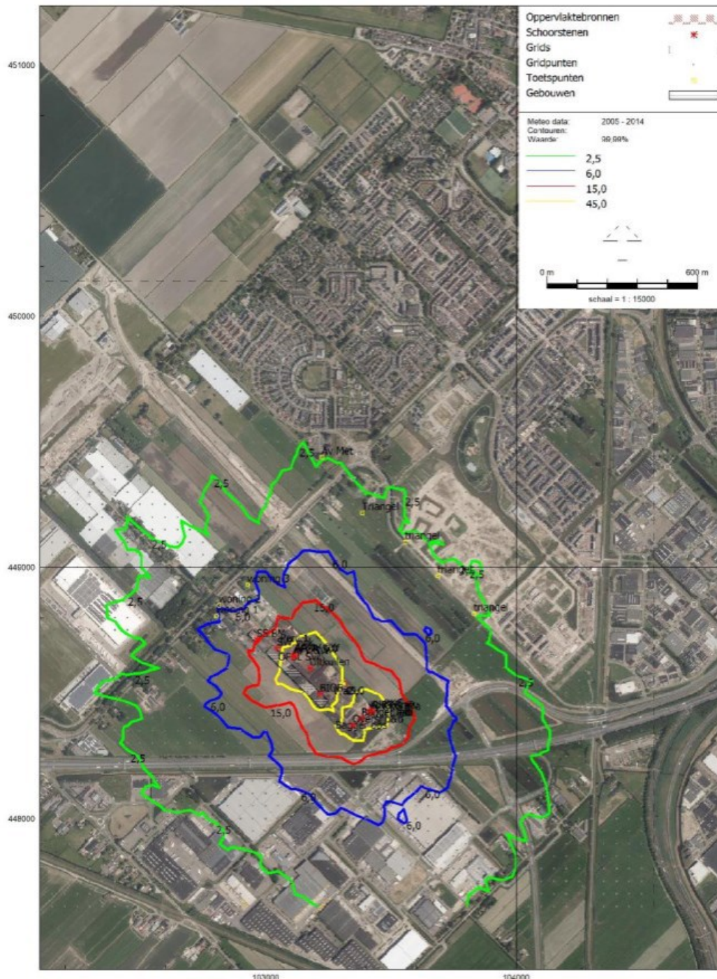
Figuur k Geurcontouren van 2,5; 7,5; 15 en 45 ou_E/m^3 als 99,99-percentielwaarde als gevolg van Waddinxveense Groenrecycling Wagro BV in de toekomstige situatie – best case ( 1.000\ ou_E/m^3 )
