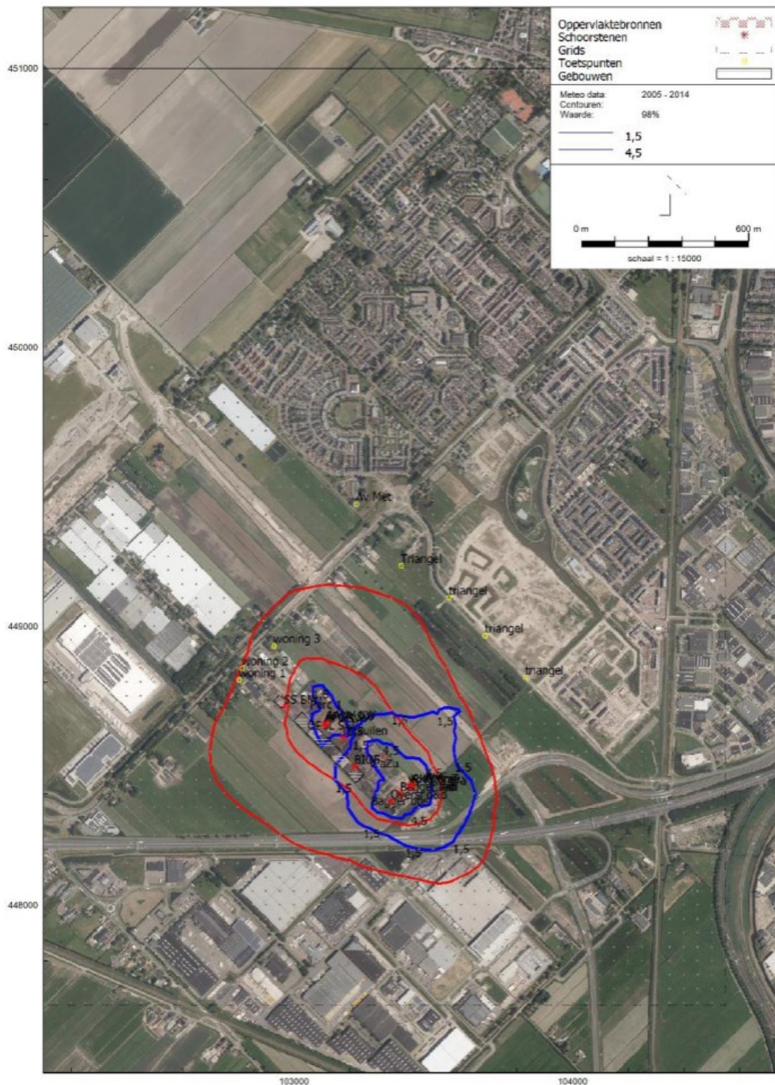
Figuur b Geurcontouren van 1,5 en 4,5 ou_E/m^3 als 98-percentielwaarde als gevolg van Waddinxveense Groenrecycling Wagro BV in de vergunde en toekomstige situatie – worst case ( 2.500\ ou_E/m^3 )
