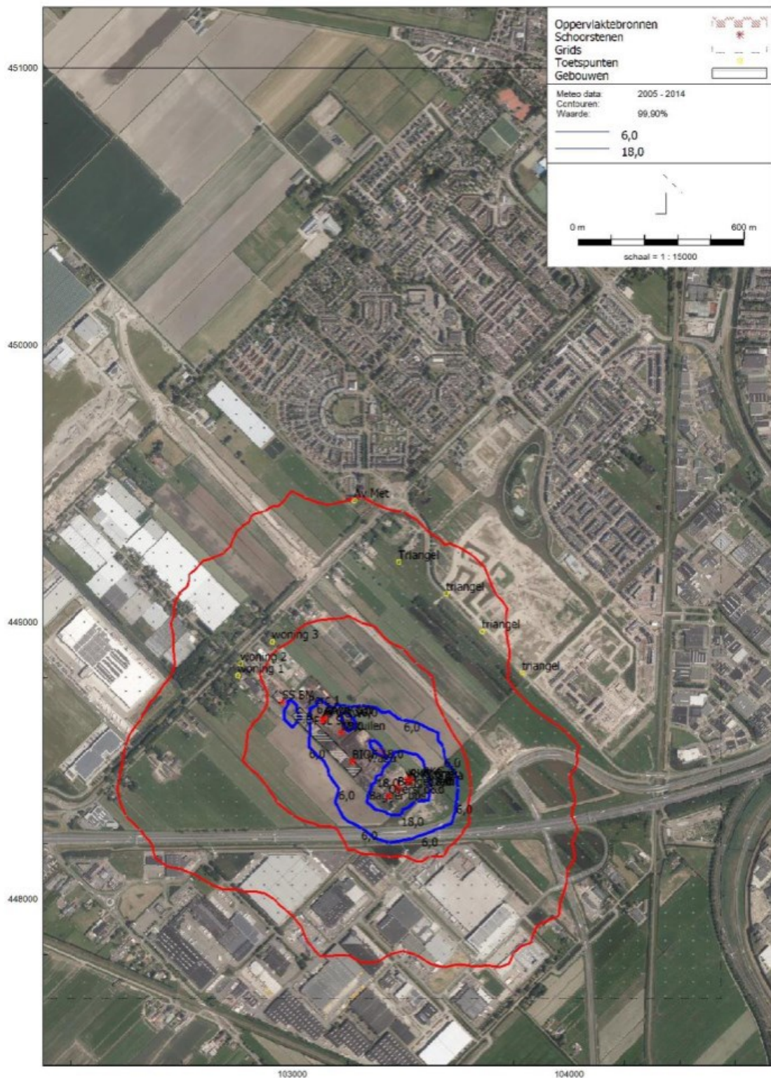
Figuur f Geurcontouren van 6 en 18 ou E /m 3 als 99,9-percentielwaarde als gevolg van Waddinxveense Groenrecycling Wagro BV in de vergunde en toekomstige situatie – worst case (2.500 ou E /m 3 )
