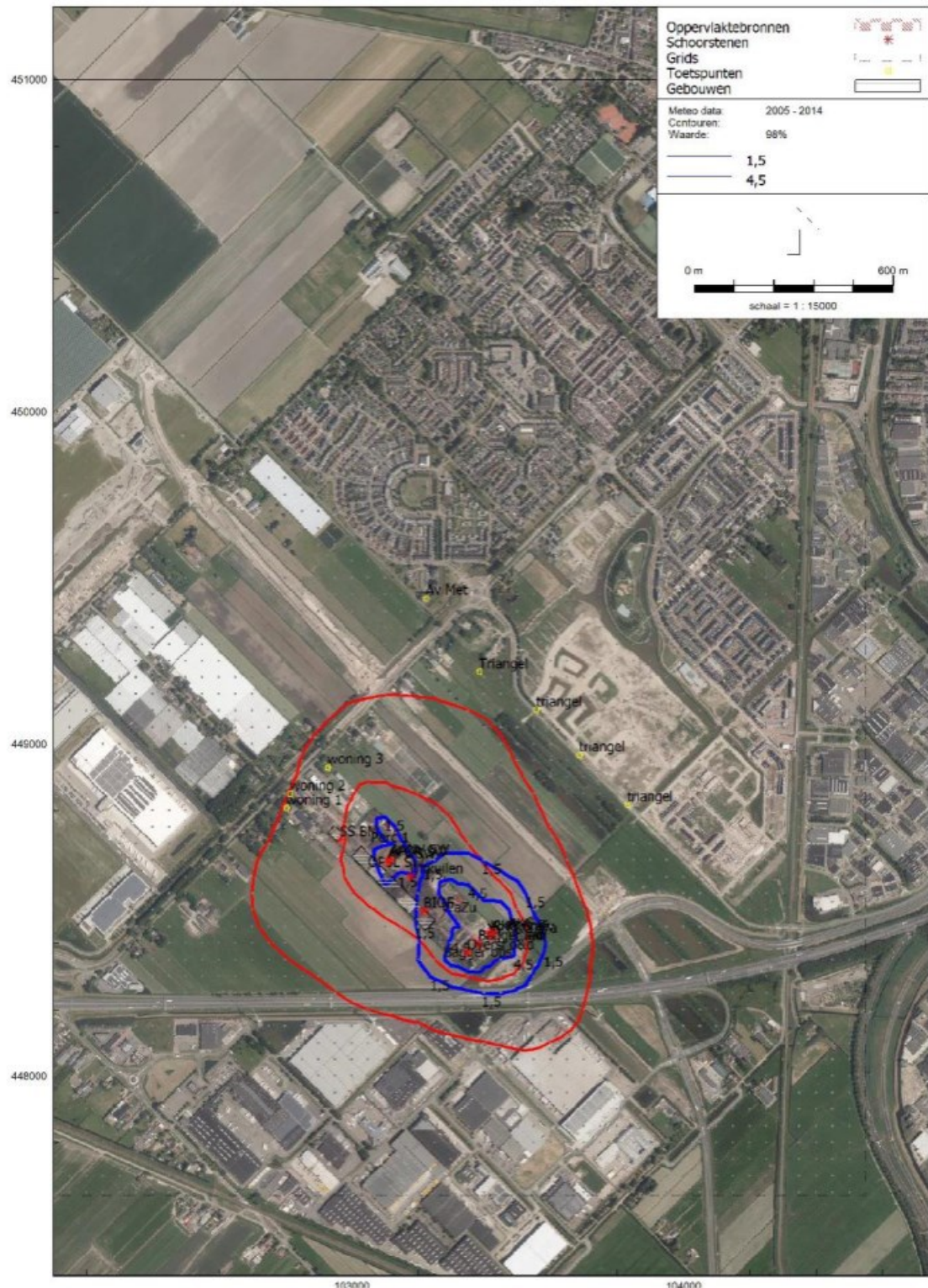
Figuur c Geurcontouren van 1,5 en 4,5 ou_E/m^3 als 98-percentielwaarde als gevolg van Waddinxveense Groenrecycling Wagro BV in de vergunde en toekomstige situatie – best case ( 1.000 \text{ ou}_E/m^3 )
