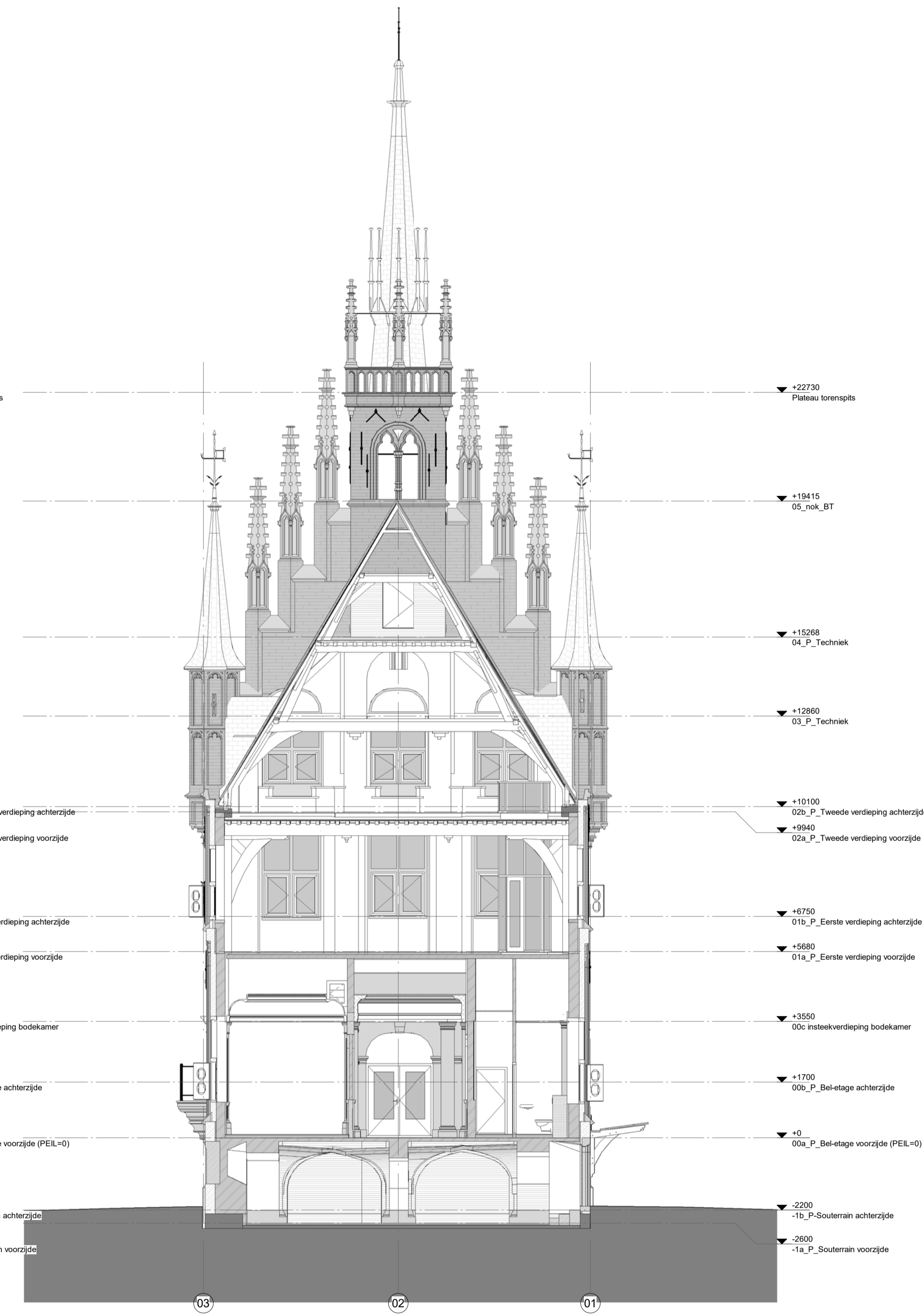
Doorsnede B-b
