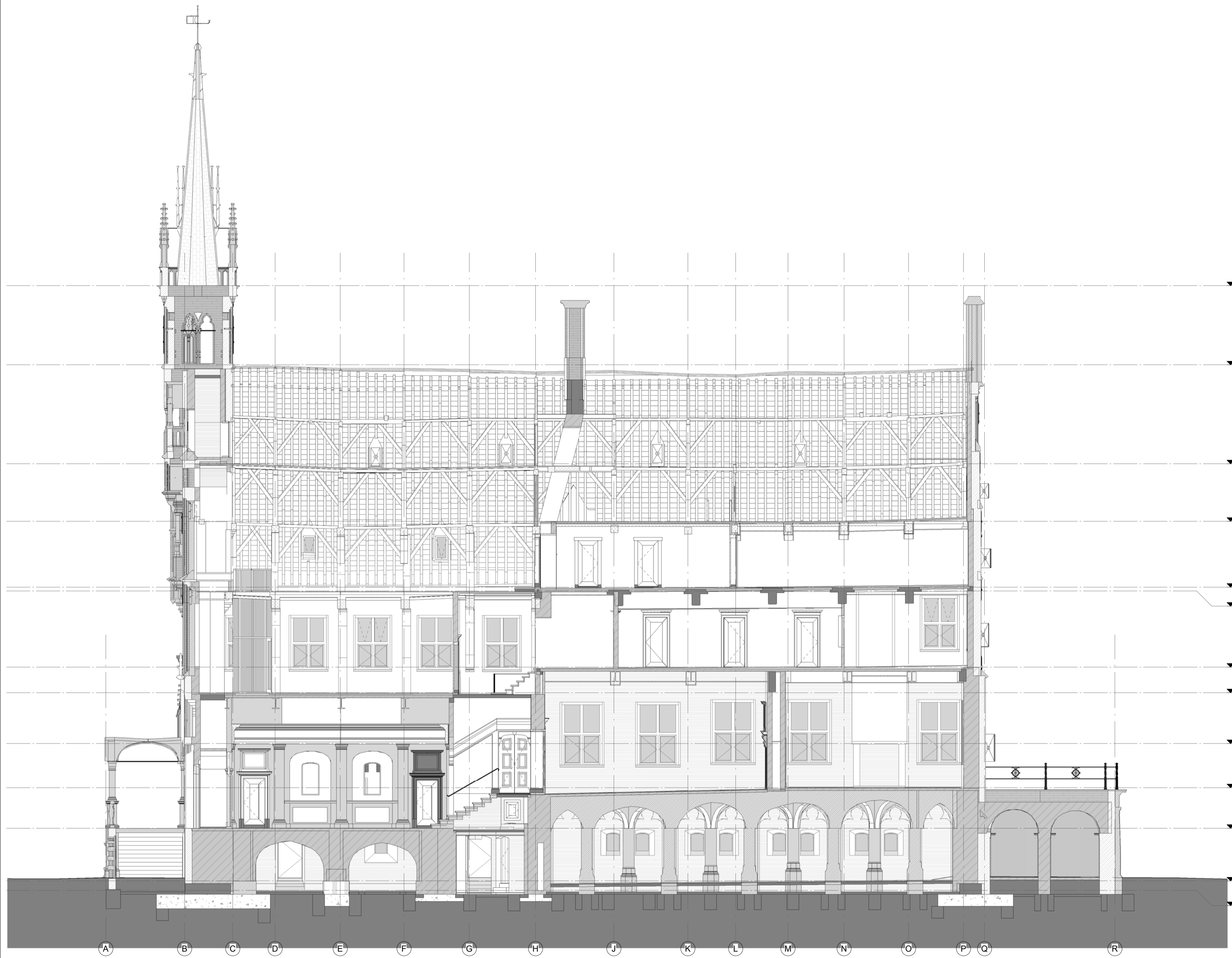
Doorsnede A-b
