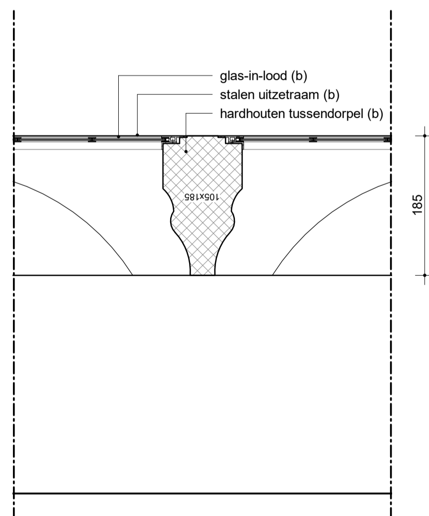
H.02b glas-in-lood (b) stalen uitzetraum (b) hardhouten tussendorpel (b)
