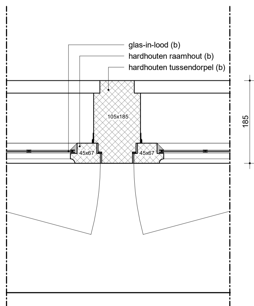
H.01b glas-in-lood (b) hardhouten raamhout (b) hardhouten tussendorpel (b)
