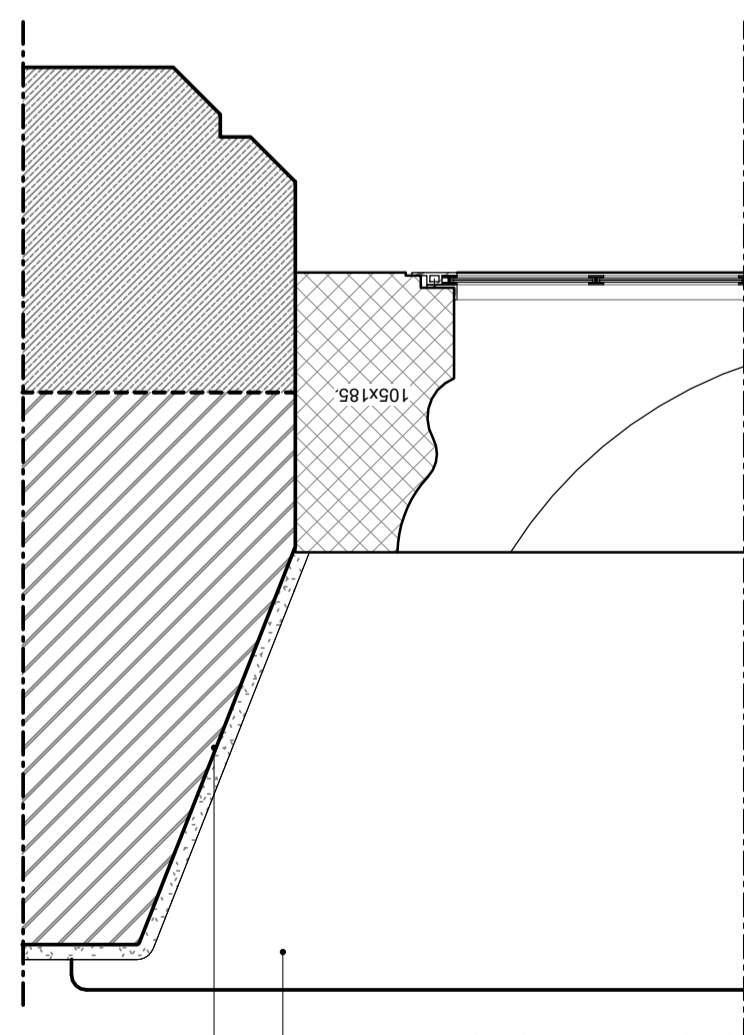
H.02a hardsteen vensterbank naaddichting
