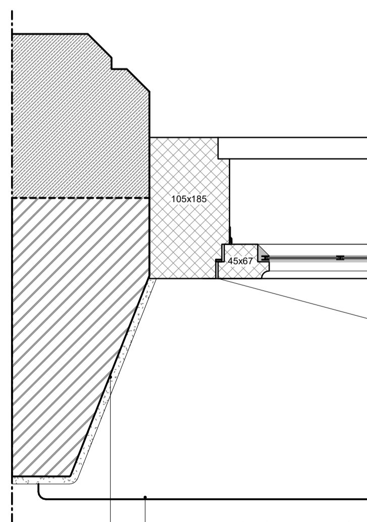
H.01a hardsteen vensterbank naaddichting
