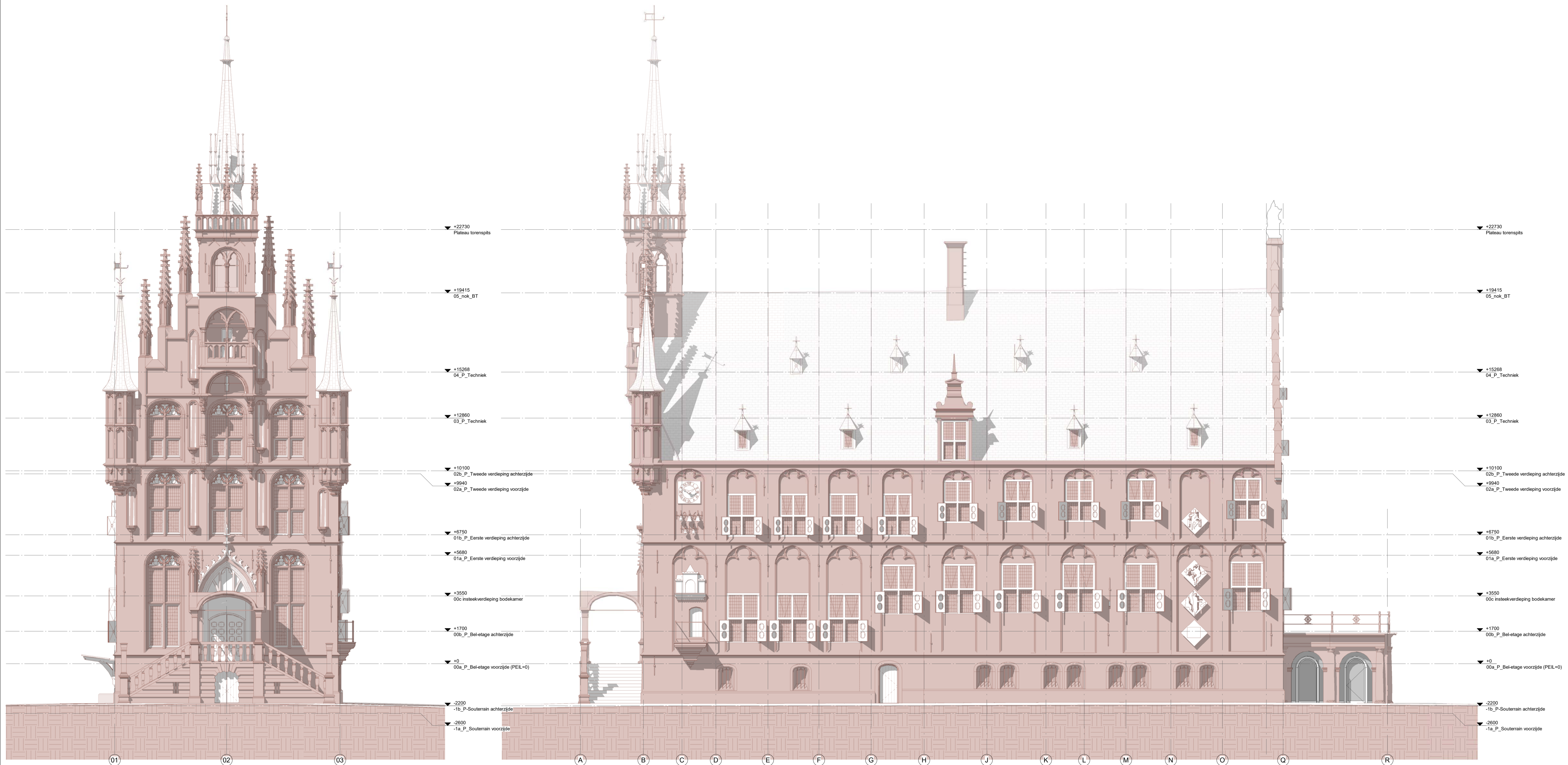
Zuidwestgevel, nieuwe toestand.
