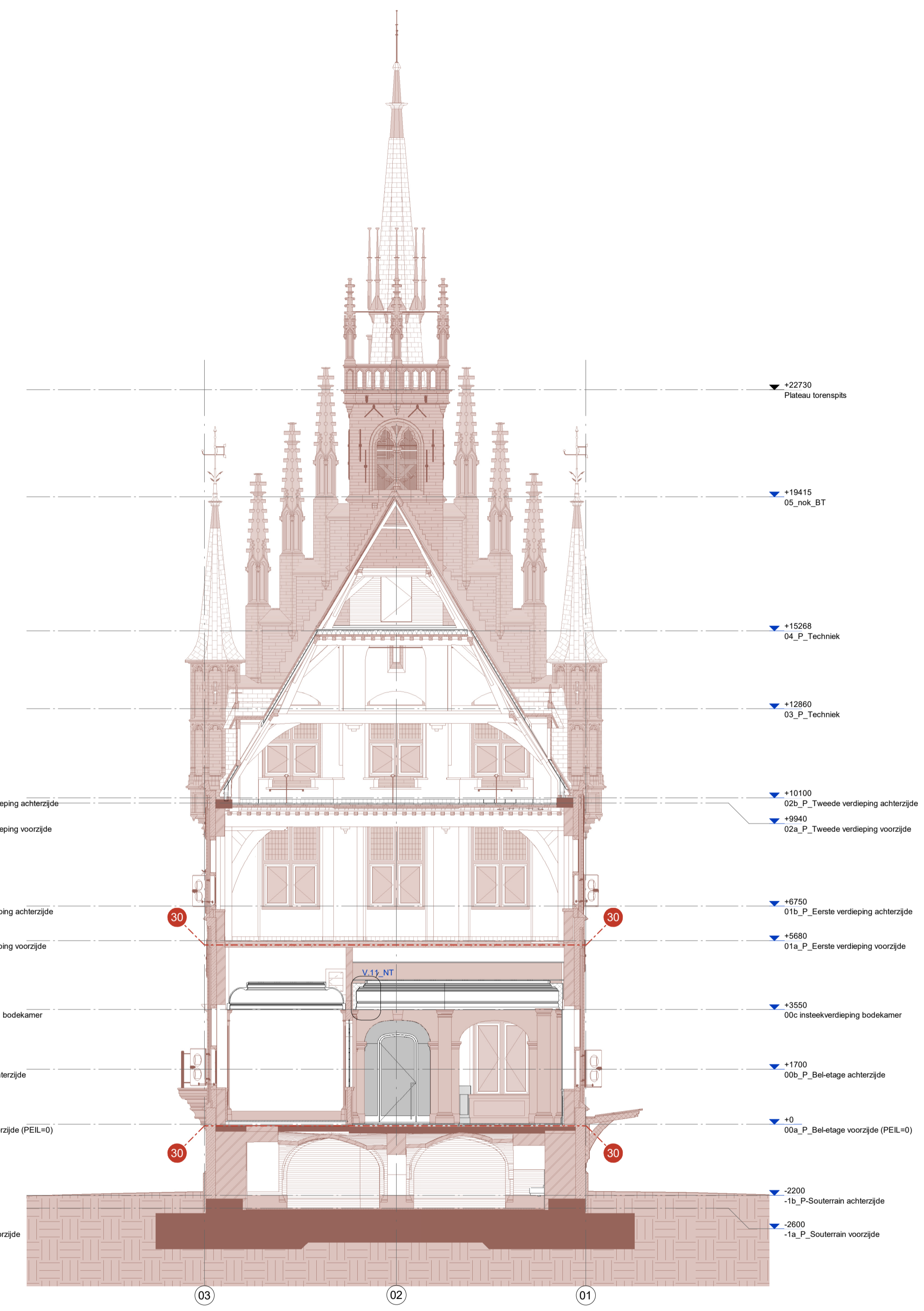
Doorsnede B-n
